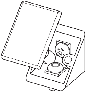
Montering av täcklock (endast för GN 30I-C-ZWSZS)
